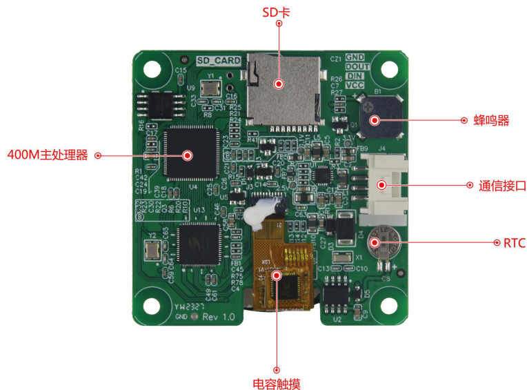
图 1-2 硬件配置图
