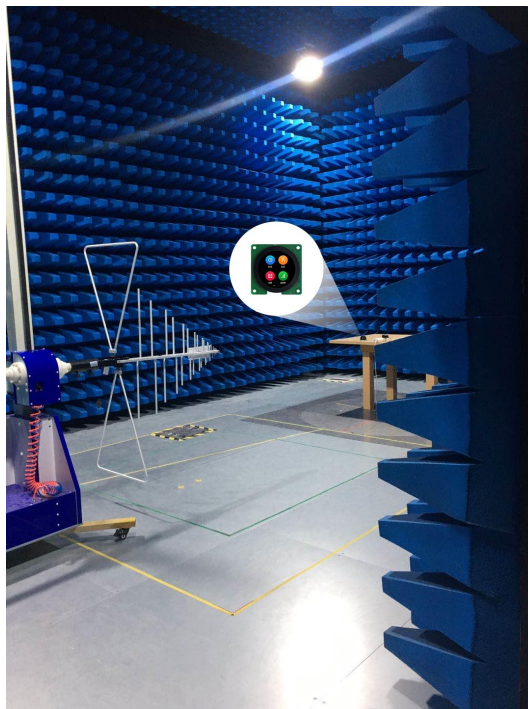
图 5-5 辐射测试图
