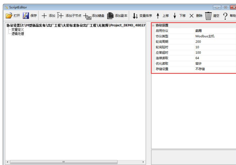
图 7-2 图 7-2 协议配置界面
