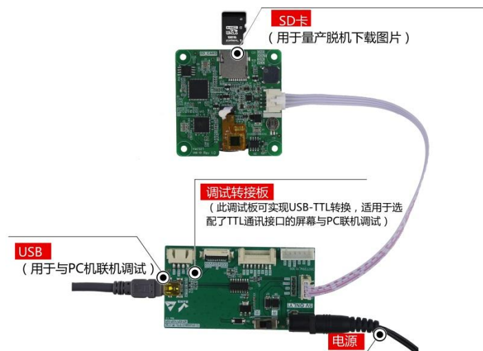
图 1-3 调试工具图
