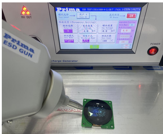
图 5-2 ESD 测试图
